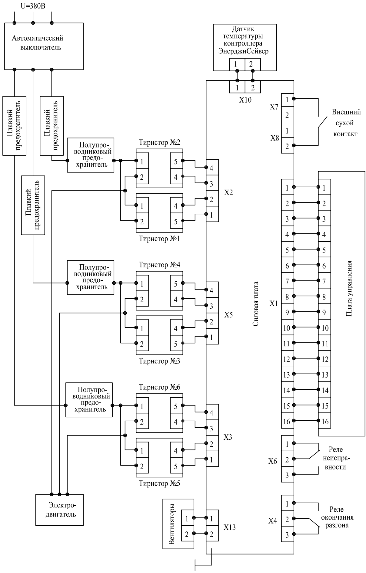
Рис. 3 Общая схема подключения контроллера ЭнерджиСейвер ES250-ES400
