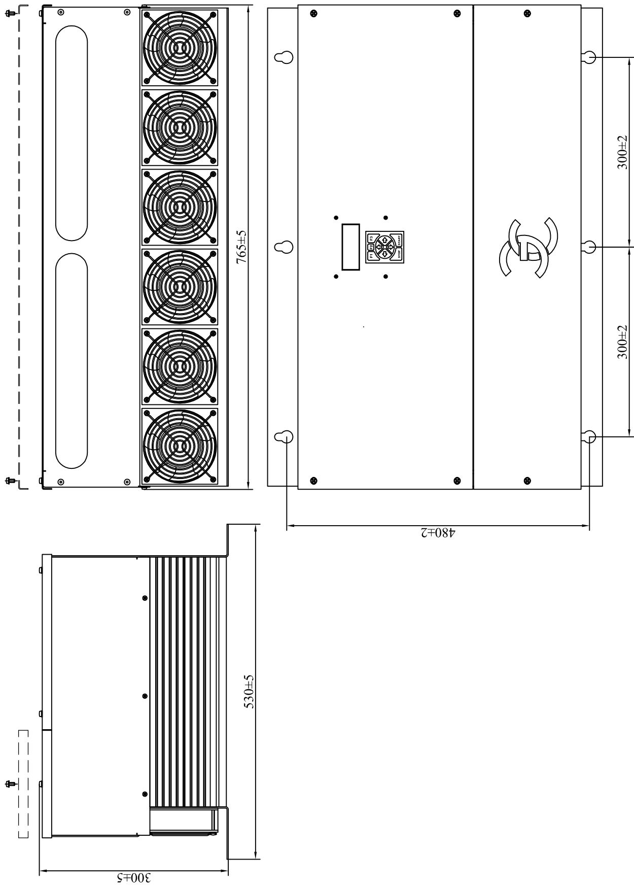
Рис. 5 Габаритные и установочные размеры контроллера ЭнерджиСейвер ES250-ES400
