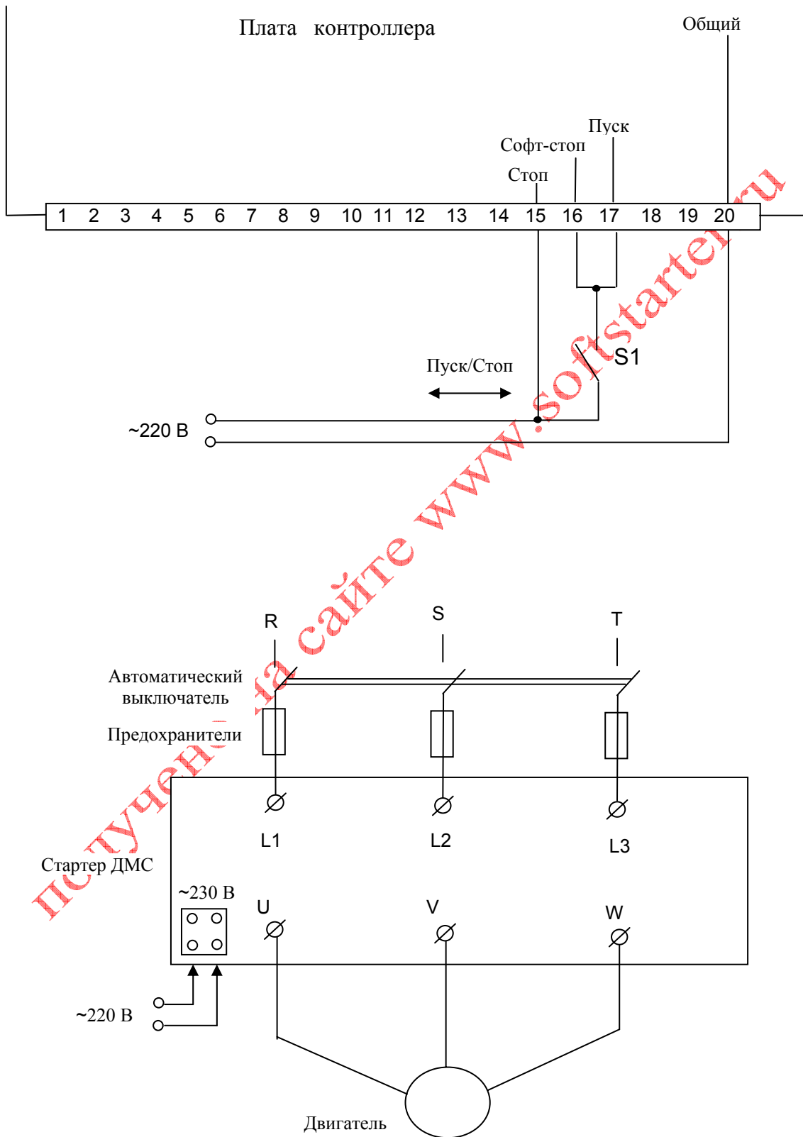
Рис. 2. Схема управления софт-стартером
